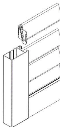
Espaceur polyamide
